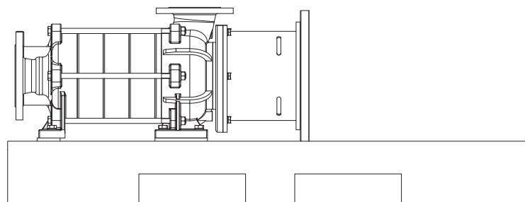
Abb. 4-4 Ausbaustufe G, Pumpe mit Magnetkupplung und Laterne, auf Grundplatte montiert
