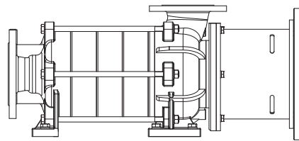
Abb. 4-3 Ausbaustufe L, Pumpe mit Magnetkupplung und Laterne
