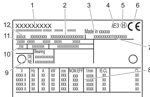
Abb. 1-4 Typenschild am Motor
