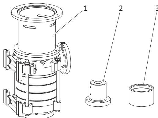
Abb. 7-3 Lieferzustand
