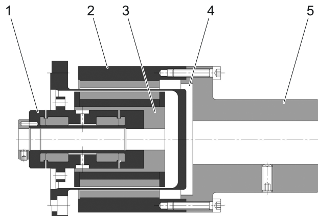
Abb. 4-2 Aufbau Magnetkupplung
