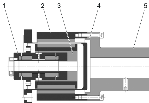
Abb. 4-2 Aufbau Magnetkupplung
