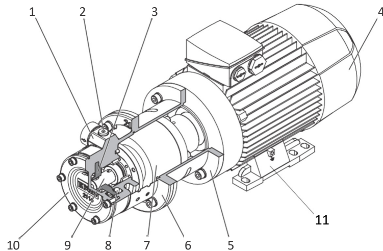
Abb. 4-1 Aufbau Pumpe
