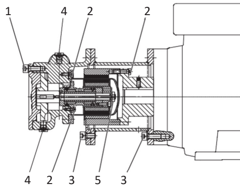
Abb. 10-1 Anziehdrehmomente PBM
