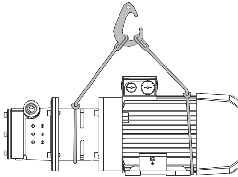
Abb. 5-1 Pumpe mit einem Kran transportieren
