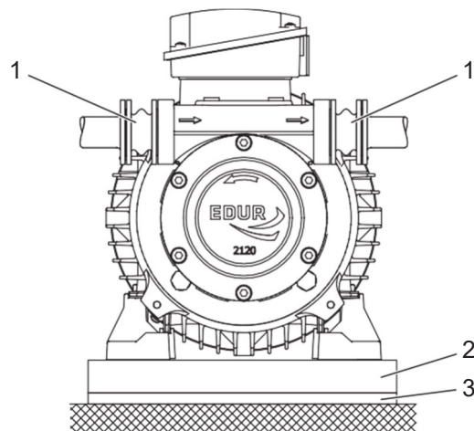
Abb. 7-2 Geräuschminimierung
